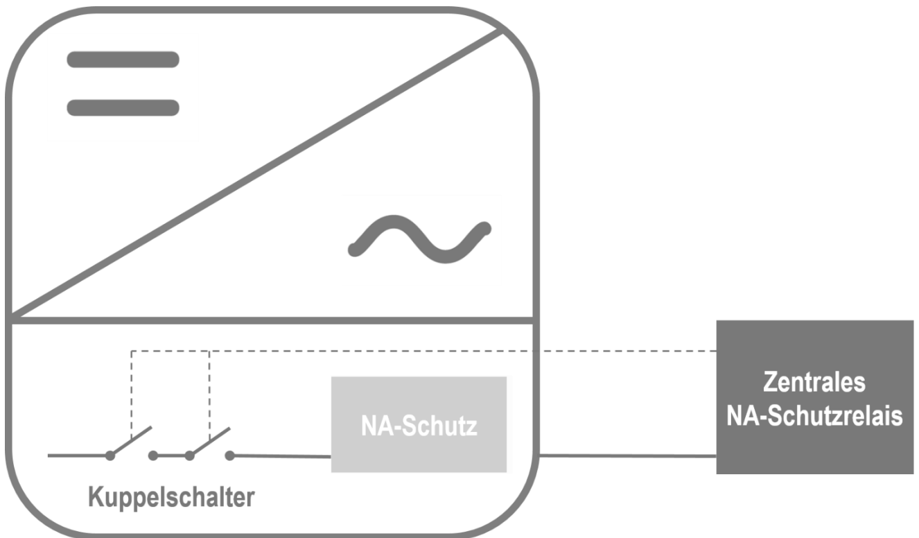
Abbildung 3: Zentrales Schutzrelais steuert Wechselrichterintegrierten Kuppelschalter
